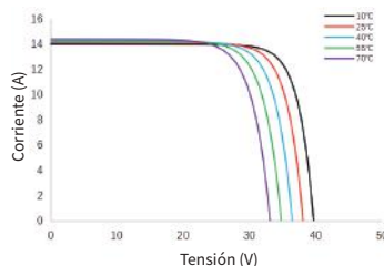
Curva de corriente- tensión SSA-48HD-445N
