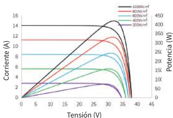
Curva de corriente/potencia-tensión SSA-48HD-445N
