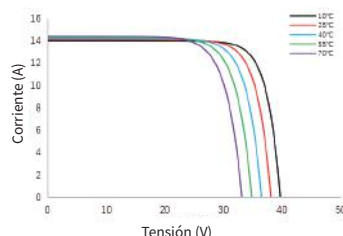
Curva de corriente- tensión SS8-54HDT-420N
