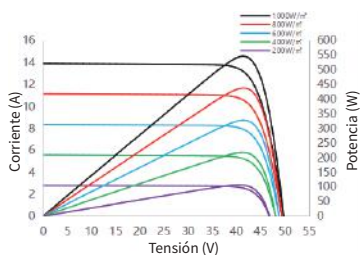
Curva de corriente/potencia-tensión SS8-72HD-545M
