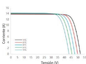
Curva de corriente- tensión SS8-72HD-545M
